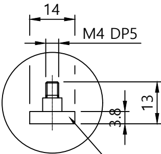
Ø14 마그네틱 자석
